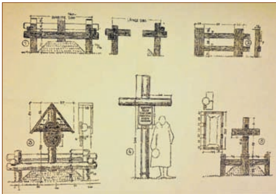
Ryc. 32. Projekty krzyży nagrobnych i cmentarnych oraz drewnianych ogrodzeń mogił autorstwa prof. Paula Bonatza
