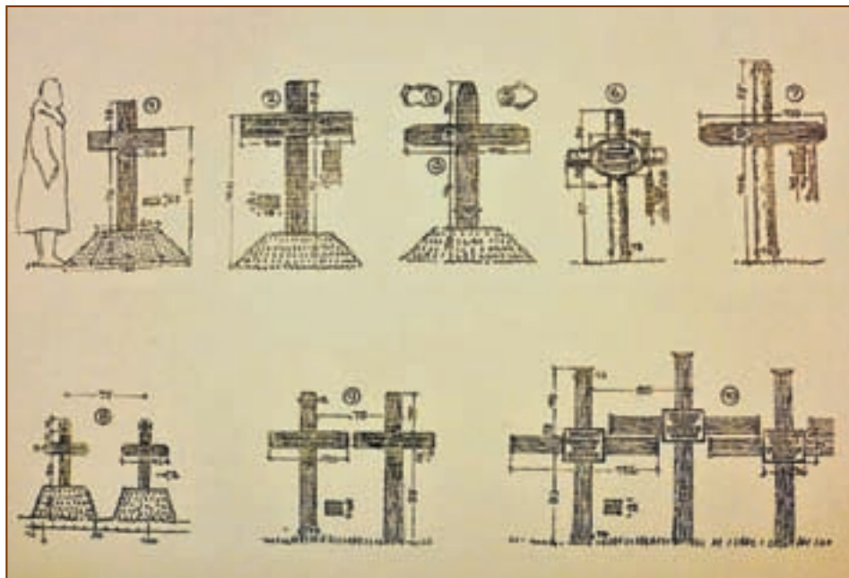
Ryc. 31. Projekty krzyży nagrobnych dla mogił jednostkowych autorstwa prof. Paula Bonatza
