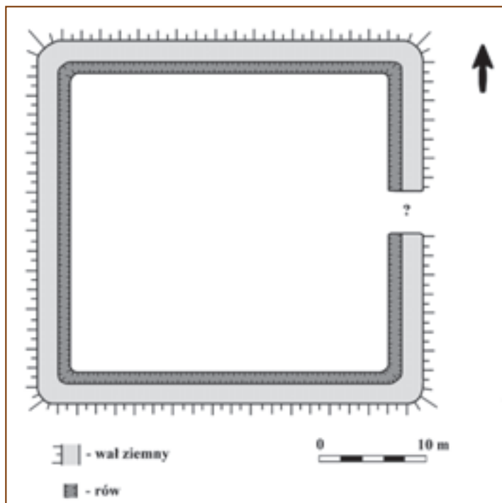
Ryc. 163. Jałówka, gm. Supraśl. Szkic współczesnego rozplanowania cmentarza wojennego. Wał ziemny i rów wyznaczające granice cmentarza są słabo zachowane, miejscami nieczytelne
