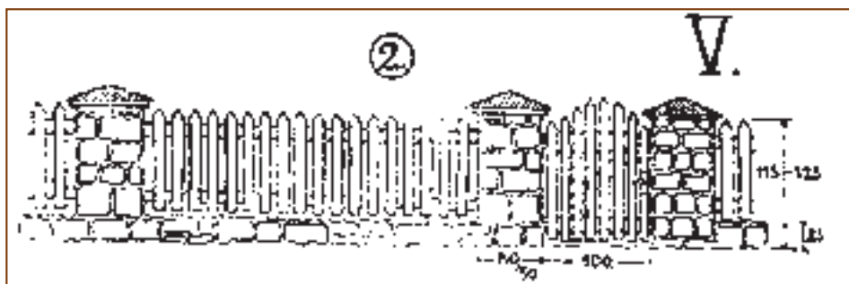
Ryc. 44. Projekt ogrodzenia cmentarza wojennego płotem z szerokich, surowych sztachet
