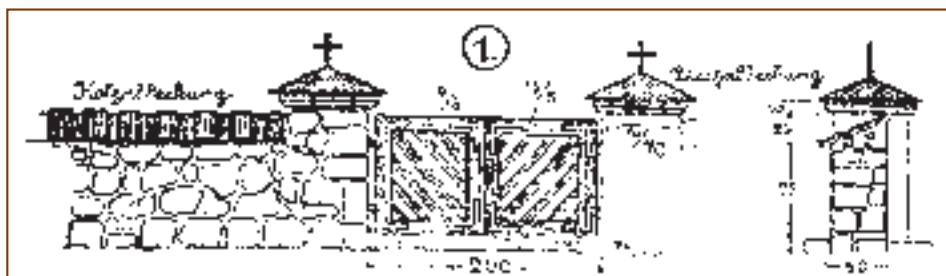
Ryc. 43. Projekt ogrodzenia cmentarza wojennego murem z kamieni polnych
