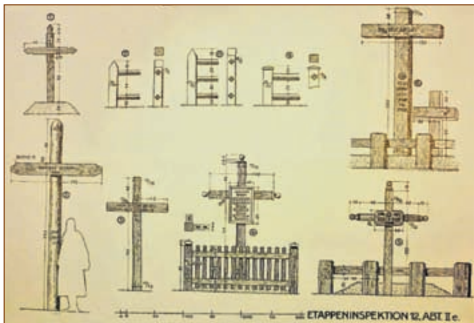
Ryc. 33. Projekty krzyży nagrobnych i cmentarnych autorstwa prof. Paula Bonatza
