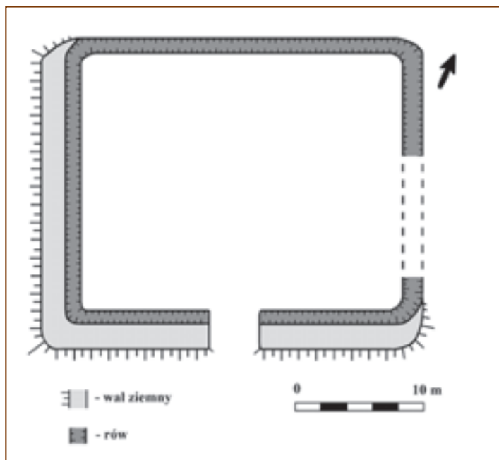
Ryc. 156. Grzybowce, gm. Gródek: Szkic współczesnego rozplanowania cmentarza wojennego. Granice nekropoli od północno-zachodu, zachodu i południa wyznacza rów i wał ziemny, od północy i północnego wschodu jedynie rów. Część wschodniej granicy cmentarza jest zniszczona
