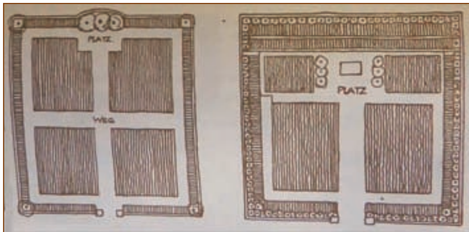
Ryc. 27. Przykłady najprostszego rozplanowania cmentarzy wojennych, uwzględniającego podział wnętrza nekropoli na pola grobowe z wyodrębnioną przestrzenią na krzyż lub pomnik
