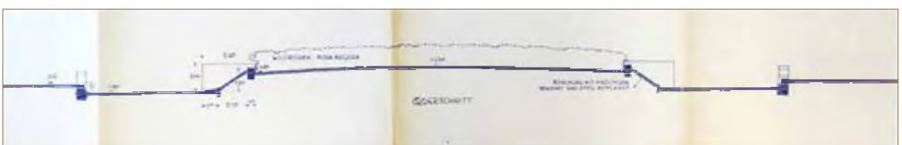
Ryc. 18. Przekrój w osi projektowanego cmentarza zbiorczego w Mogilach-Dębowej (projekt) (Źródło: PA AA, sygn. 48012 [Volksbund Deutsche Kriegsgräberfürsorge e.V. an das Auswärtige Amt. Anlage. Berlin, 16.4.35]).
