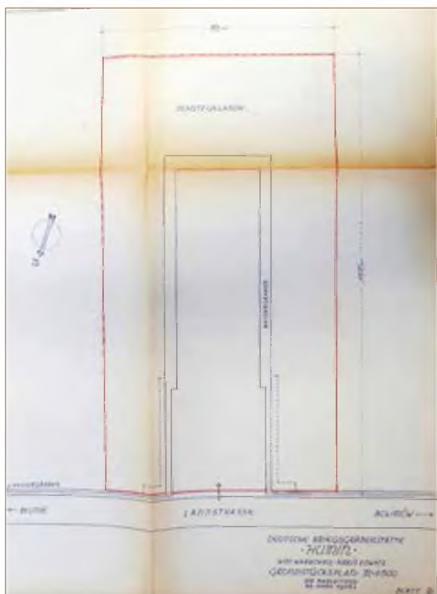
Ryc. 27. Projekt zagospodarowania terenu cmentarza w Huminie z zaznaczoną planowaną strefą ochronną (Źródło: PA AA, sygn. 48012 [Volksbund Deutsche Kriegsgräberfürsorge e.V. an der Deutsche Botschaft Warschau, 5. Februar 1936]).
